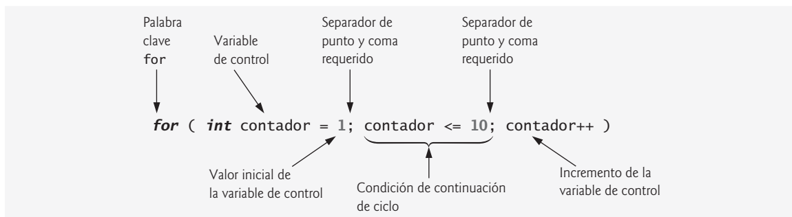
Figura 6.3 | Componentes del encabezado de la instrucción for .
