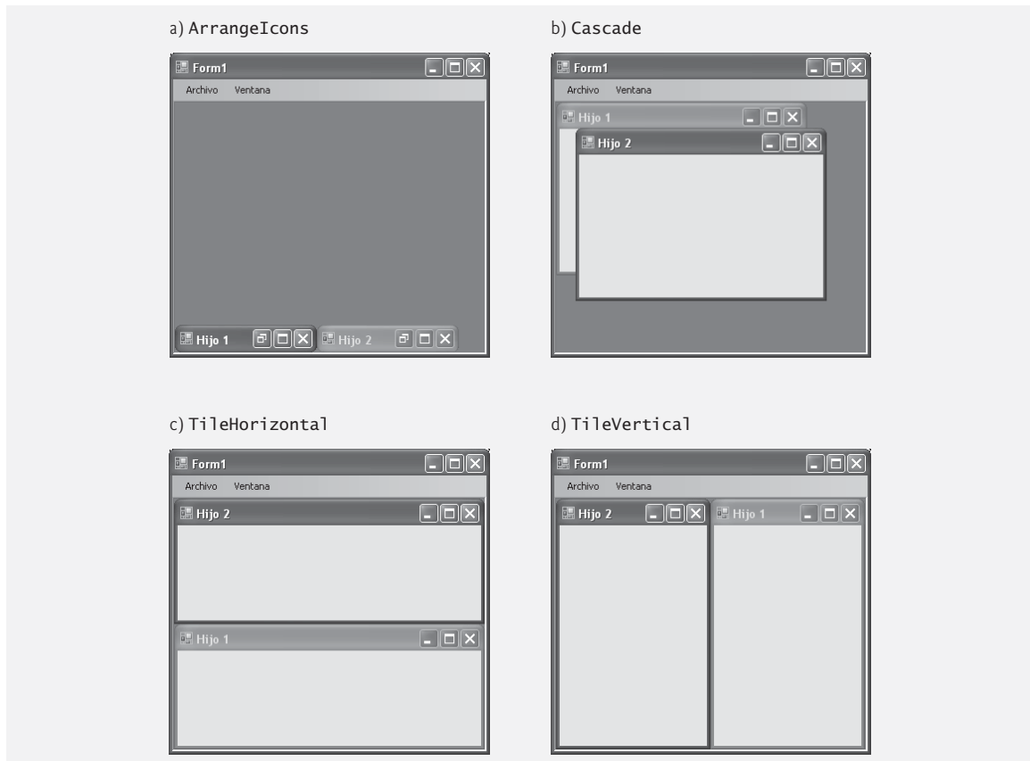
Figura 14.42 | Valores de la enumeración MdiLayout .
