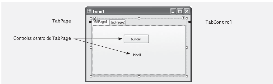
Figura 14.33 | Ejemplo de un control TabControl con objetos TabPage .
