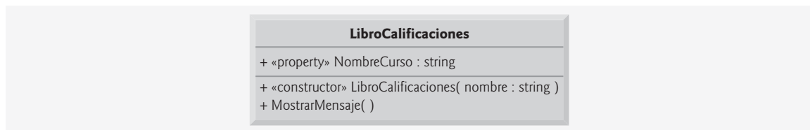
Figura 4.14 | Diagrama de clases de UML donde se indica que la clase LibroCalificaciones tiene un constructor con el parámetro Name del tipo string .
