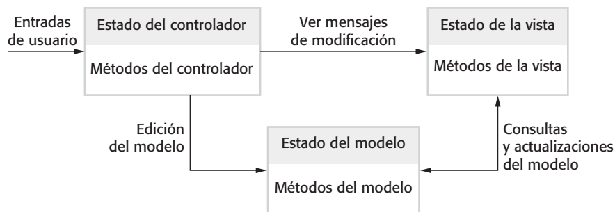
Figura 16.5 Patrón Modelo-Vista-Controlador
